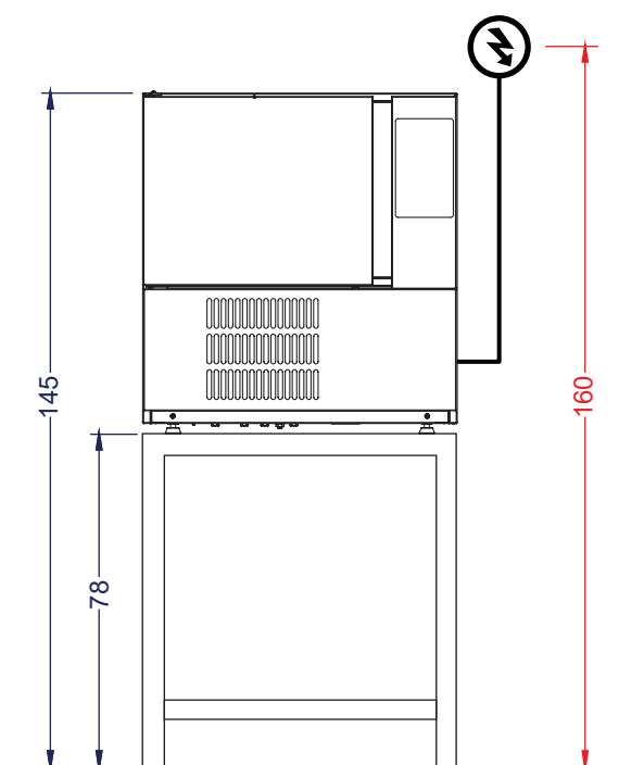
Vista Elevación
