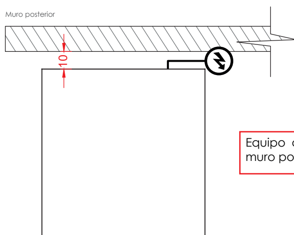
Vista Planta
