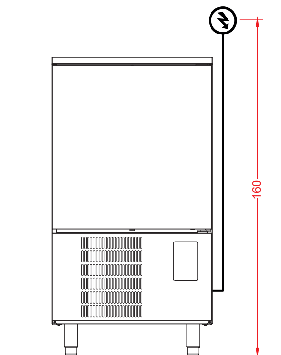
Vista Elevación
