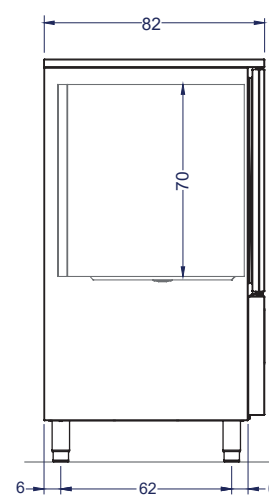
Vista Izquierda
