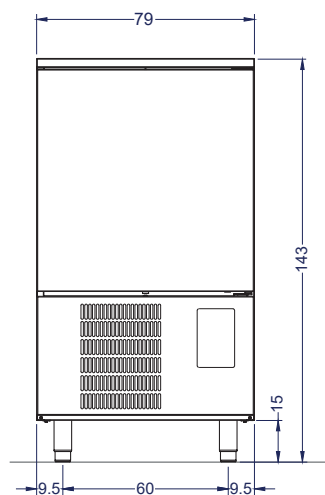
Vista Elevación
