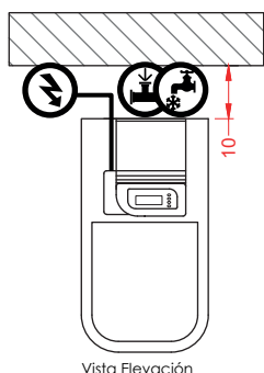
Vista Elevación
