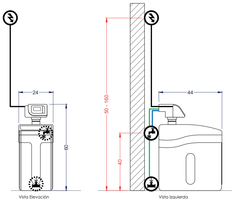
Vista Elevación
