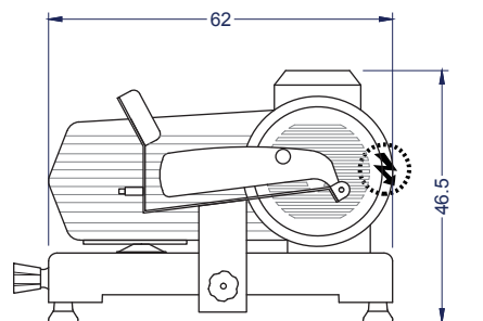
Vista Elevación
