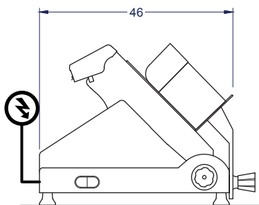
Vista Izquierda
