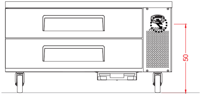
Vista Elevación
