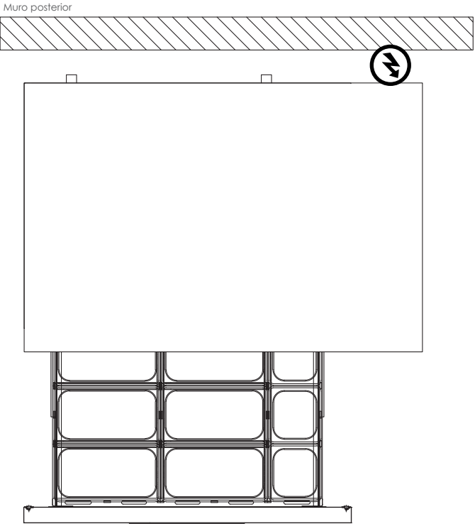
Vista Planta
