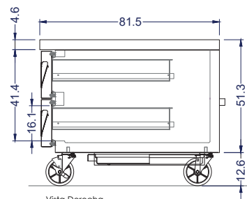
Vista Derecha
