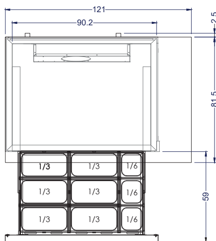
Vista Planta
