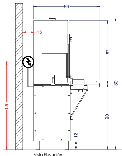
Vista Elevación
