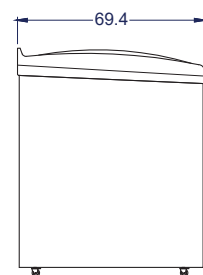
Vista Izquierda
