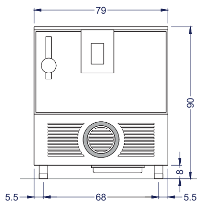
Vista Elevación
