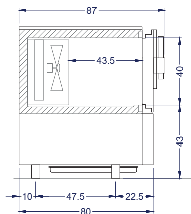
Vista Izquierda
