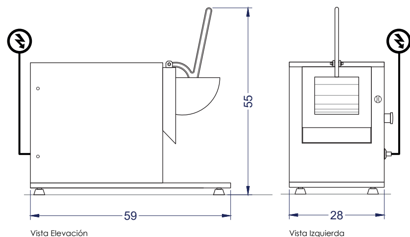
Vista Elevación
