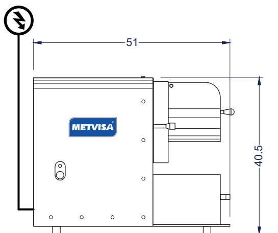
Vista Elevación
