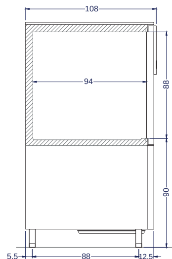
Vista Izquierda
