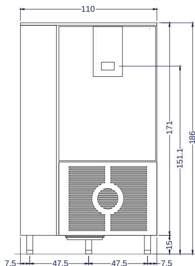
Vista Elevación
