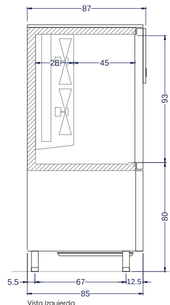
Vista Izquierda
