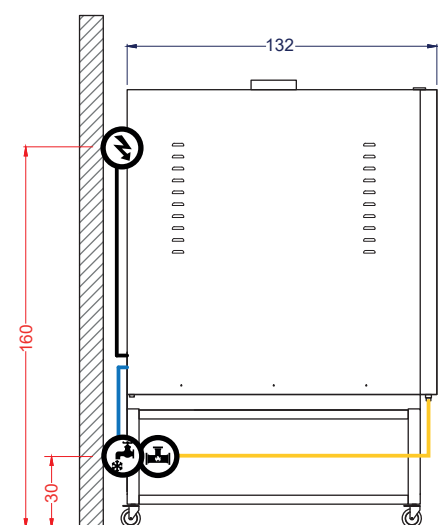
Vista Izquierda
