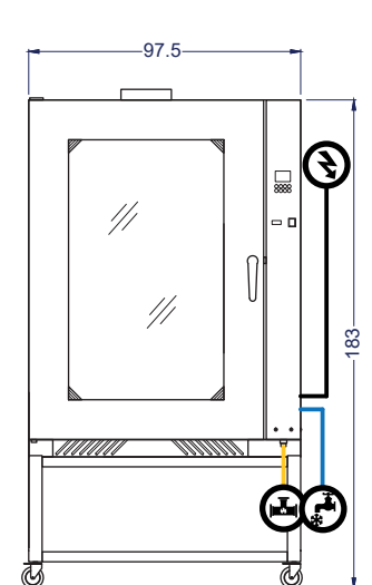
Vista Elevación
