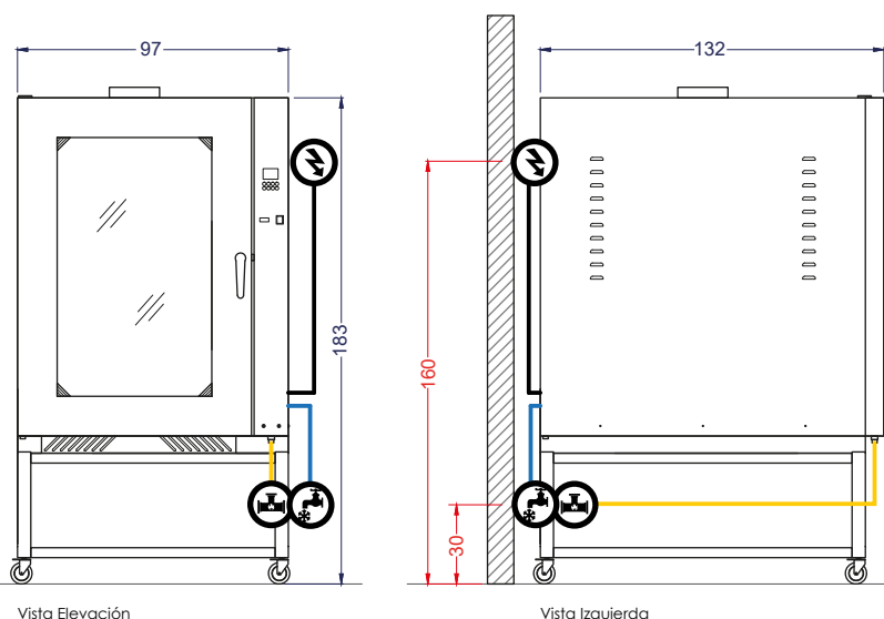
Vista Elevación
