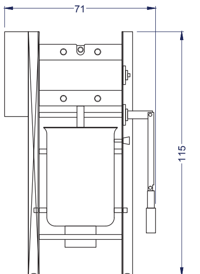
Vista Elevación
