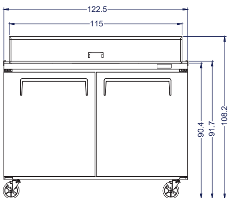
Vista Elevación
