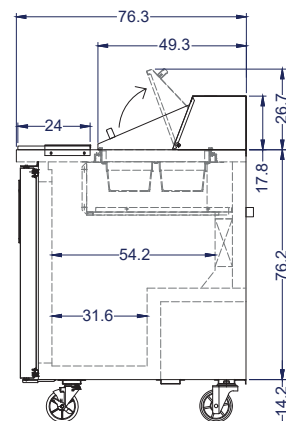
Vista Derecha
