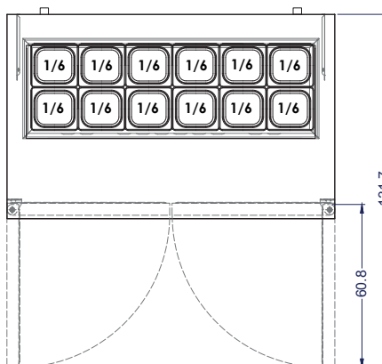
Vista Planta
