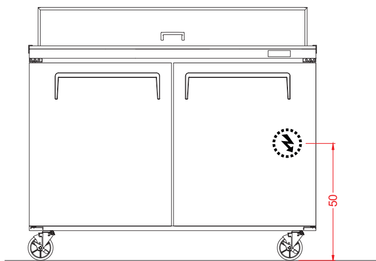
Vista Elevación
