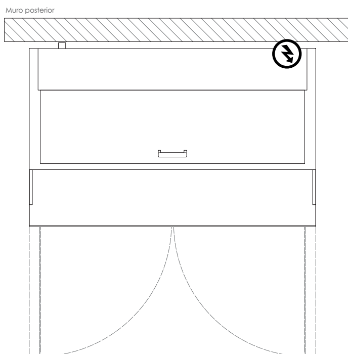
Vista Planta
