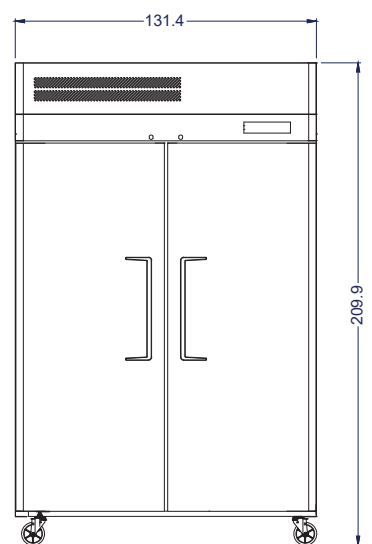
Vista Elevación
