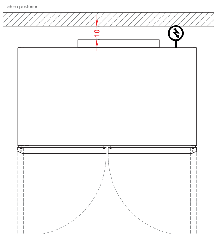
Vista Planta
