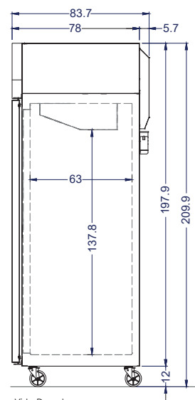
Vista Derecha
