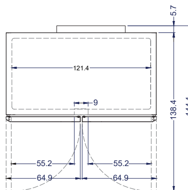
Vista Planta
