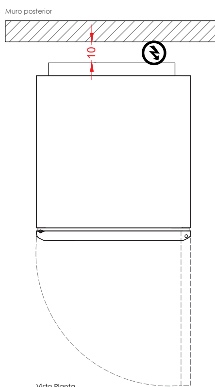
Vista Planta
