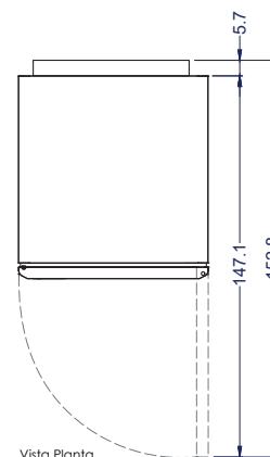
Vista Planta
