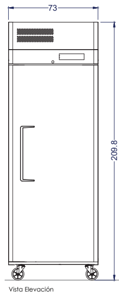
Vista Elevación
