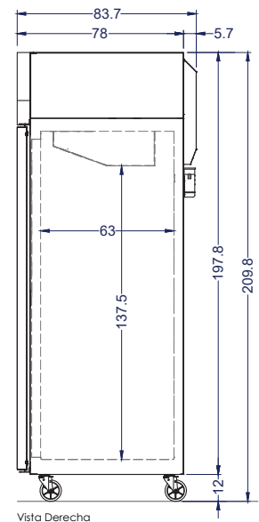
Vista Derecha
