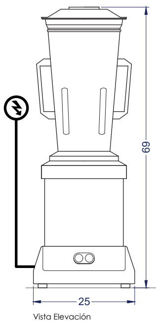
Vista Elevación
