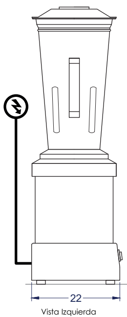
Vista Izquierda
