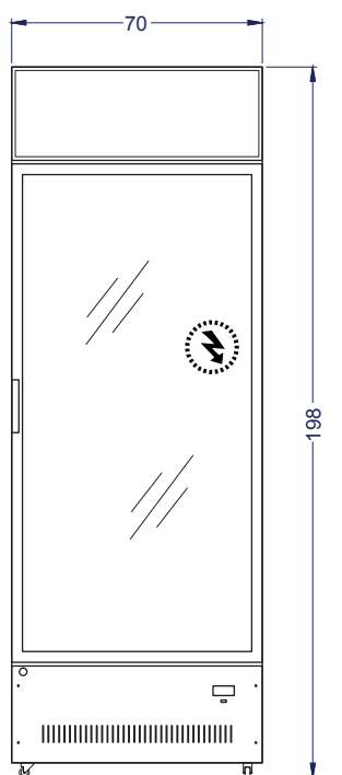
Vista Elevación
