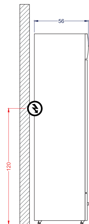
Vista Izquierda
