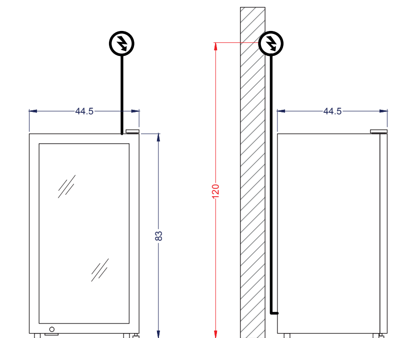
Vista Elevación
