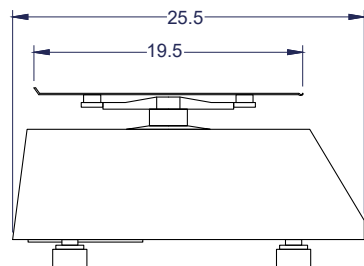
Vista Izquierda
