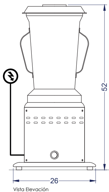
Vista Elevación
