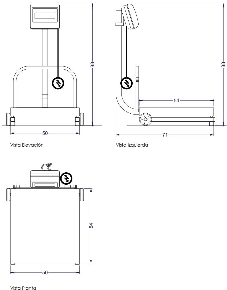
Vista Planta
