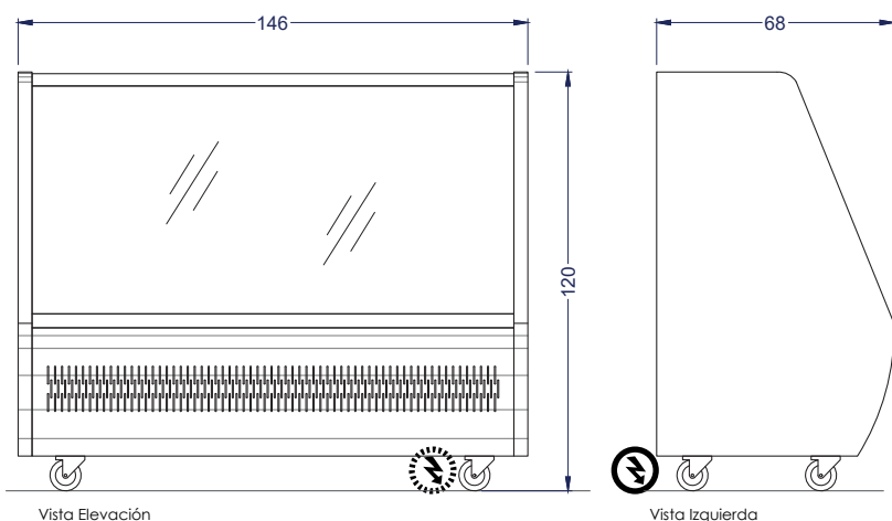
Vista Elevación
