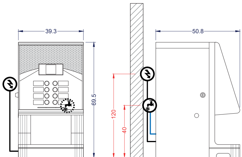
Vista Elevación
