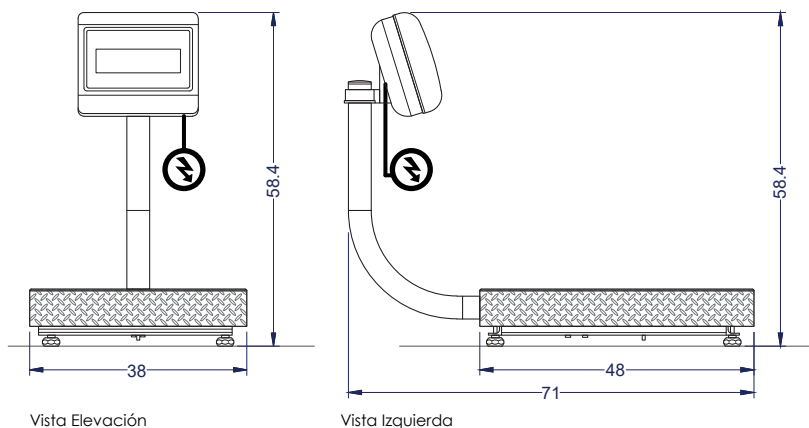
Vista Elevación
