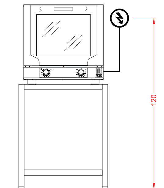
Vista Elevación
