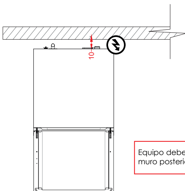
Vista Planta
