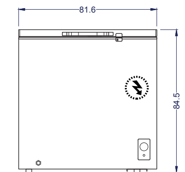
Vista Elevación
