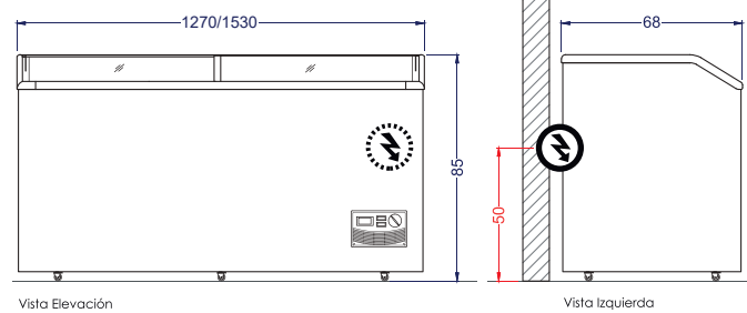
Vista Elevación
