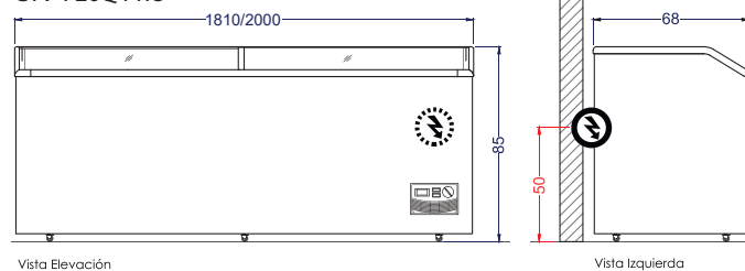
Vista Elevación
