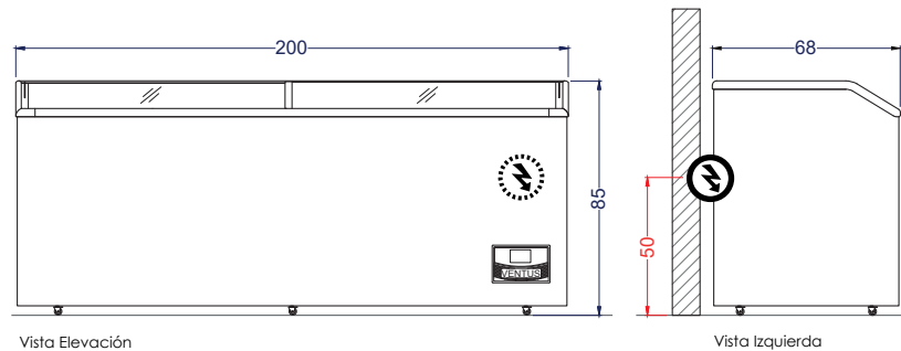
Vista Elevación
