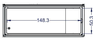
Vista Planta
