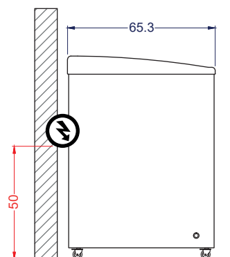
Vista Izquierda
