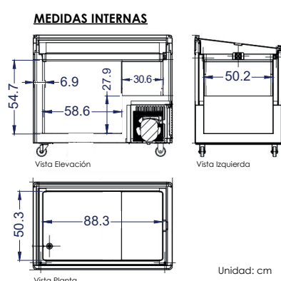
Vista Planta
