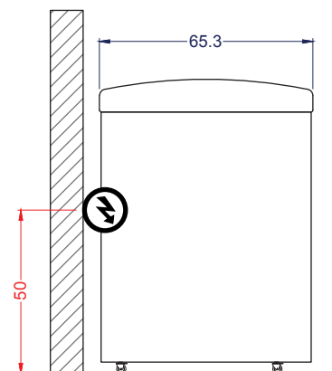
Vista Izquierda
