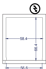
Vista Planta
