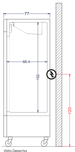
Vista Derecha
