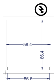
Vista Planta
