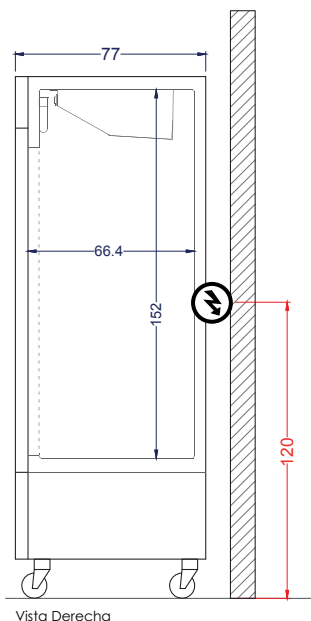
Vista Derecha
