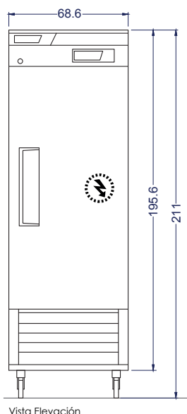
Vista Elevación
