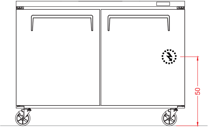
Vista Elevación
