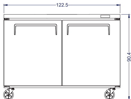
Vista Elevación
