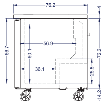
Vista Derecha
