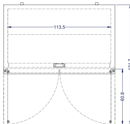
Vista Planta
