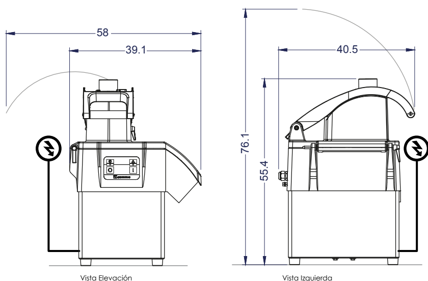
Vista Elevación
