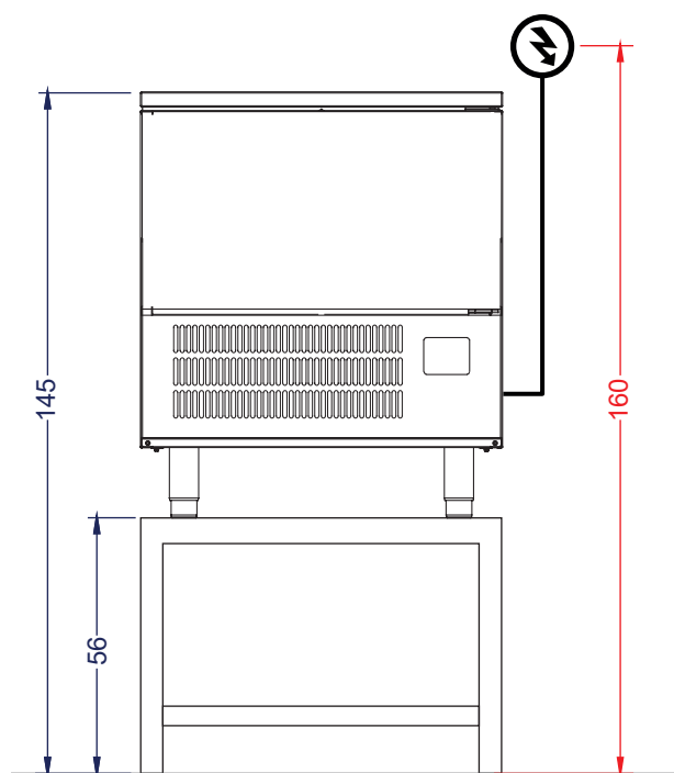
Vista Elevación
