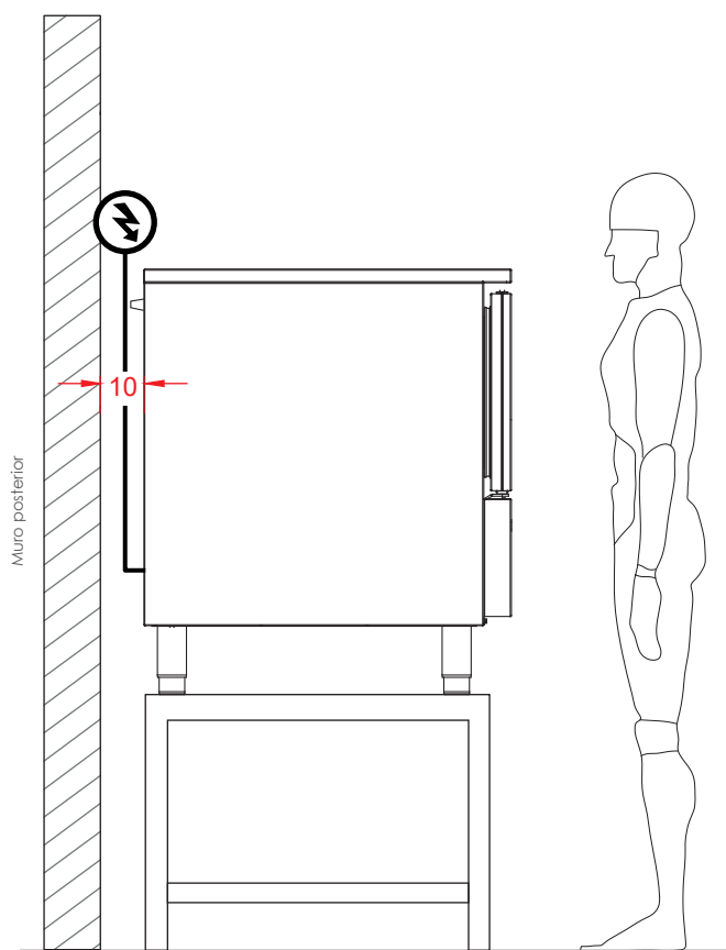
Vista Izquierda
