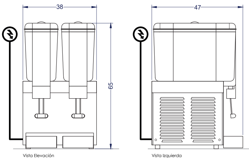
Vista Elevación
