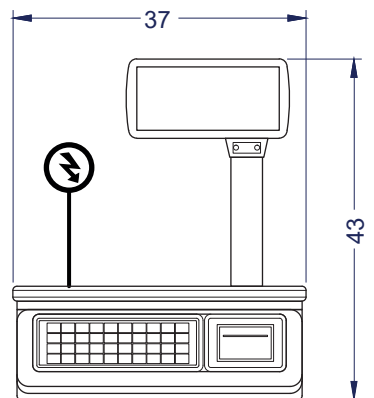
Vista Elevación
