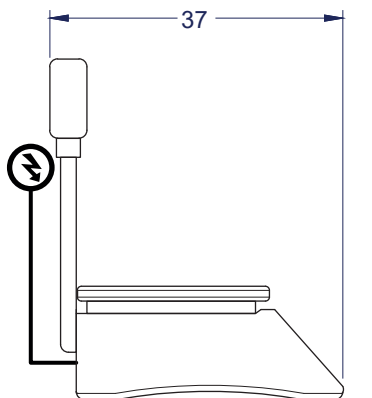
Vista Izquierda
