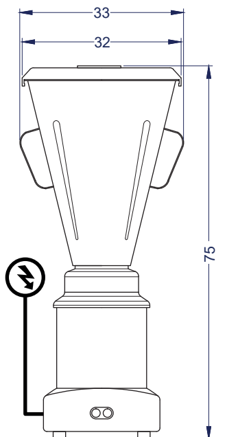
Vista Elevación
