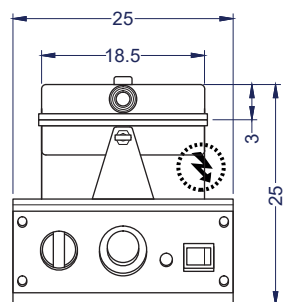
Vista Elevación
