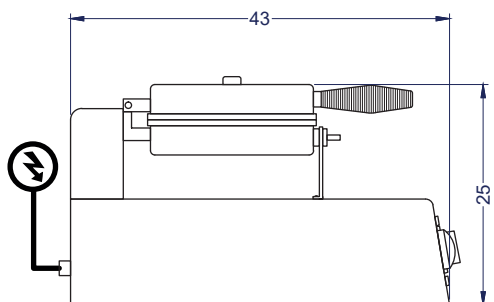
Vista Izquierda
