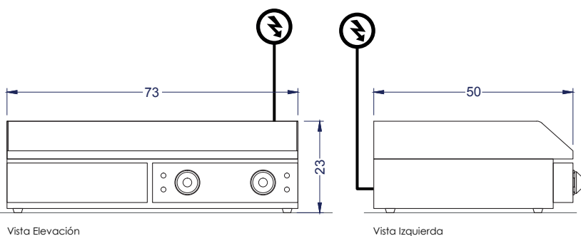
Vista Elevación
