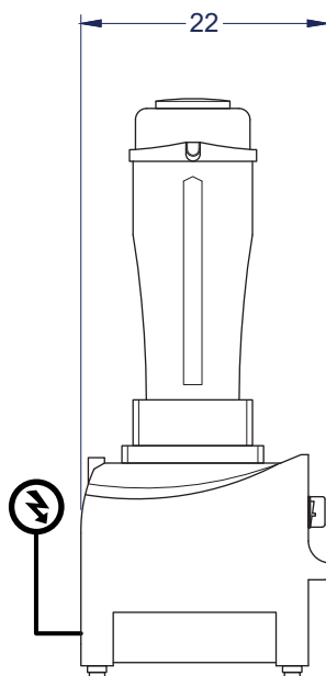
Vista Izquierda
