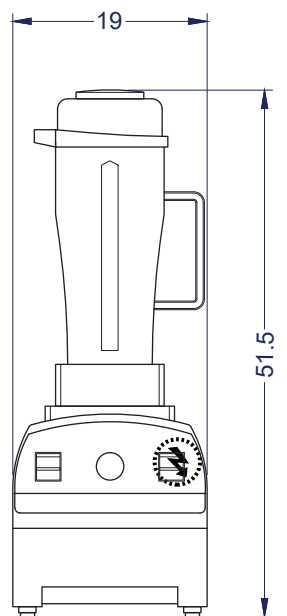
Vista Elevación
