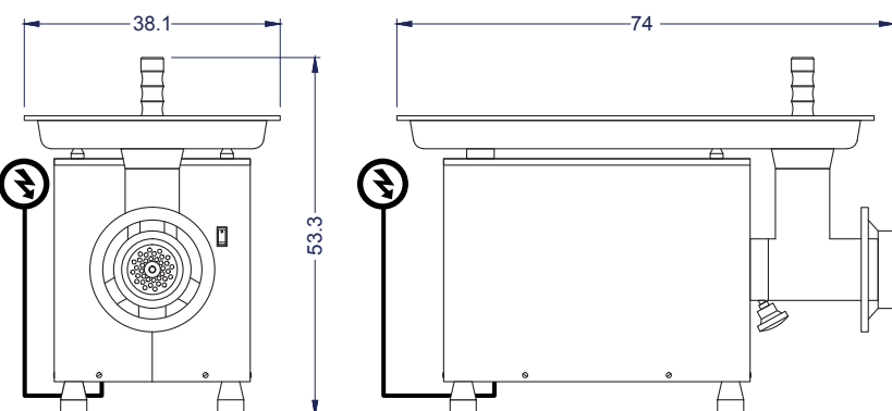
Vista Elevación
