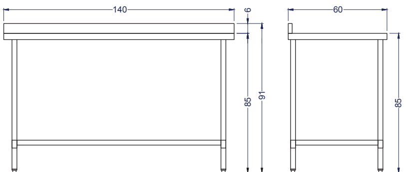
Vista Elevación
